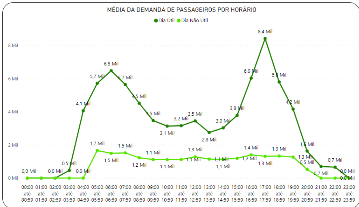
Gráfico 3-80 Demanda Horária – Santa Cruz – dez/2023
