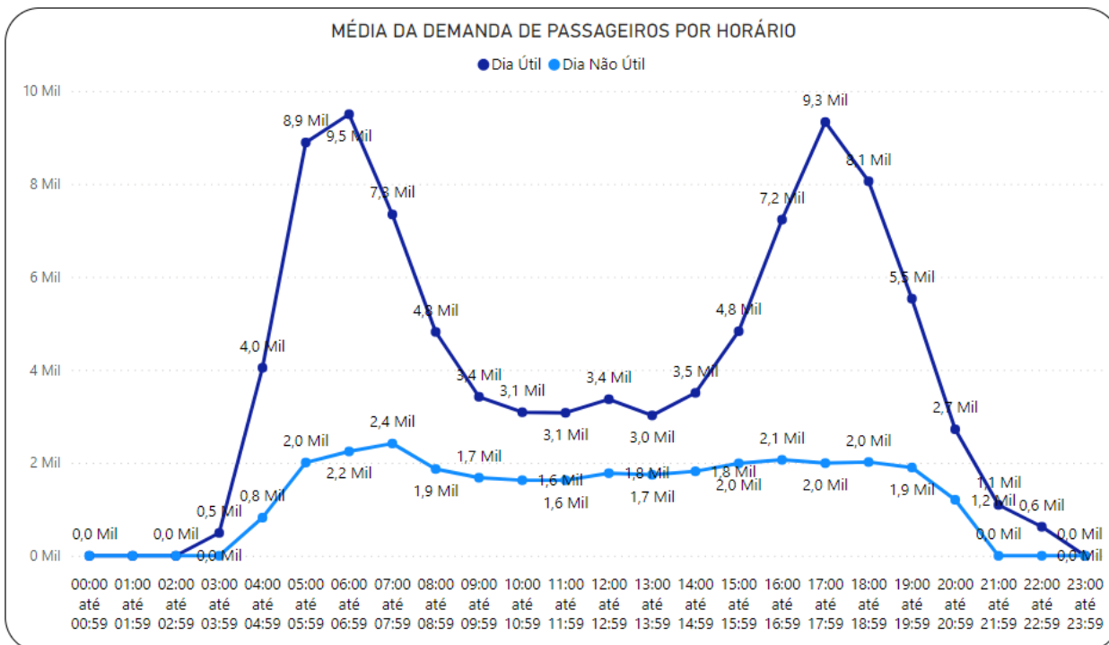
Gráfico 3-79 Demanda Horária – Japeri – dez/2023
